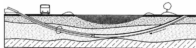
Rys.3) Przeciąganie rurociągu
