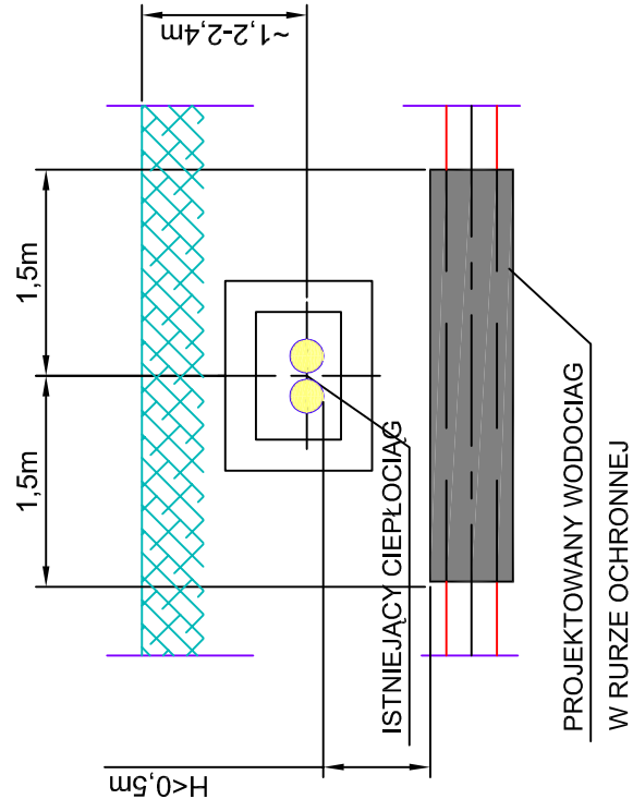
SZCZEGÓŁ WYKONANIA ZABEZPIECZENIA 1:50
