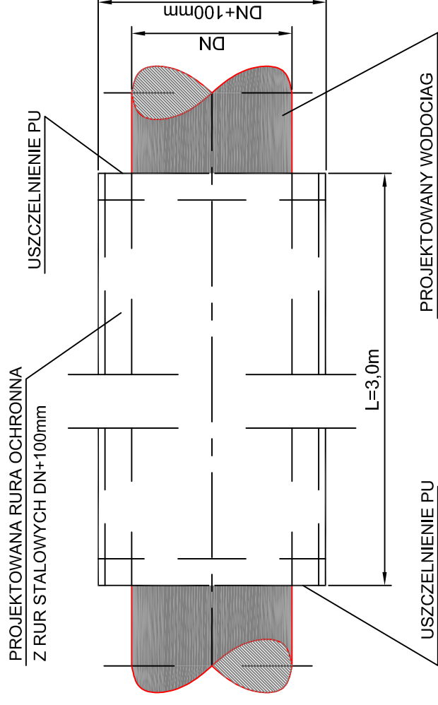
SZCZEGÓŁ RURY OCHRONNEJ
